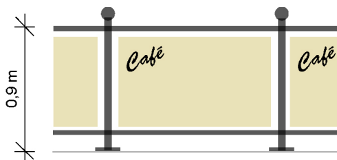
Beskrivning som visar utseende och höjd på ett kafés avgränsning (staket).
